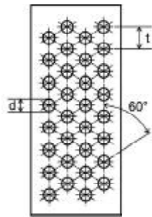
Abb. 1 Rundlochung in versetzten Reihen Fig. 1 Trous ronds en lignes alternantes
