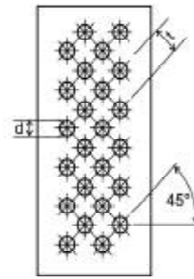
Abb. 2 Rundlochung in diagonal versetzten Reihen Fig. 2 Trous ronds en lignes diagonalement alternantes
