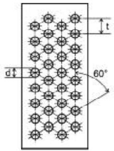
III.1 Round hole perforation in offset lines Fig. 1 Fori rotondi in disposizione faltata
