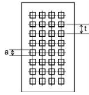
III.2 Square hole perforation in straight lines Fig. 3 Fori quadrati in disposizione rettilinea
