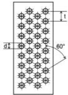
III. 1 Round hole perforation in offset lines Fig. 1 Fori rotondi in disposizione faltata
