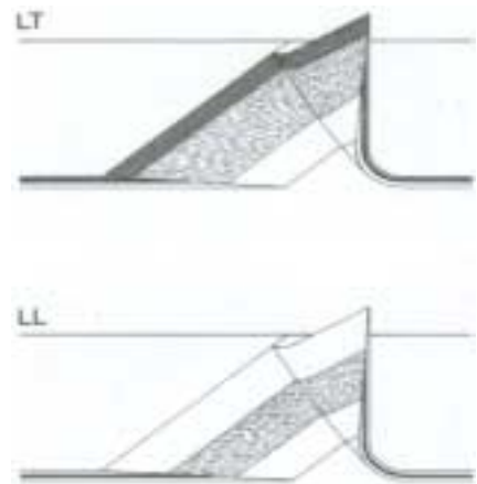
Pict. 3 Construction of flat belts / Fig. 3 Costruzione delle cinghie
